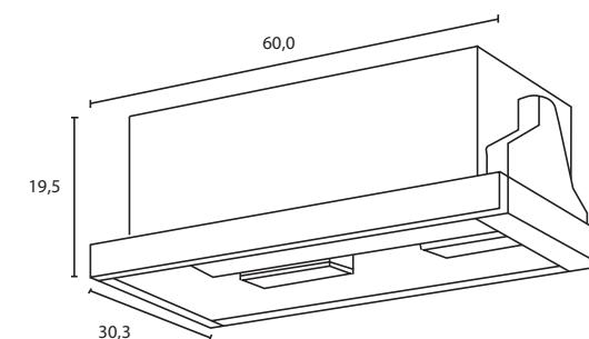
Dimensión de instalación Medidas en cm
