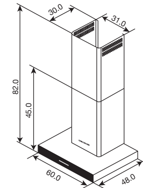
Dimensión de instalación Medidas en cm
